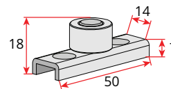
ART.1587 ROLLER GUIDE
